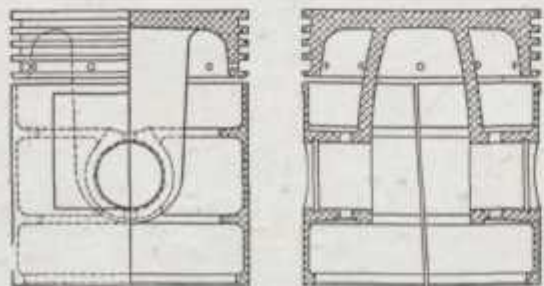
La caractéristique du piston Ray-Day en alliage d'aluminium est un mode de compensation de la dilatation. La chemise du piston est sectionnée en un point comme le montre la figure et est entièrement séparée du fond qui porte les segments, sauf deux longs bossages qui retiennent la chemise au fond. La distance entre ces bossages a été déterminée soigneusement de façon que la dilatation du fond du piston entre les supports des bossages soit égale à la dilatation du cylindre en fonte; de cette façon le piston s'ajuste exactement dans le cylindre, à froid et à chaud.
