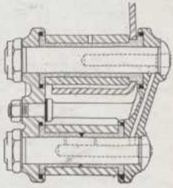
Pour éviter l'introduction de la boue et de corps étrangers, les douilles des lamelles de ressorts sont pourvues de rondelles de feutre comme le montre la figure, et, pour offrir une grande surface d'appui aux charges latérales, elles sont munies de larges collerettes aux extrémités. La rondelle de cuir en forme de V représentée au centre de la douille inférieure est destinée à empêcher les fuites d'huile.
