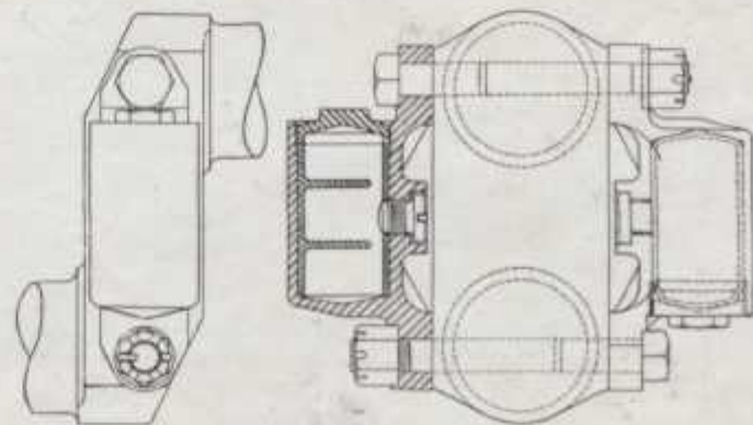
L'amortisseur de vibration consiste en deux cartouches remplies aux 94 centièmes de mercure et fixées de part et d'autre de la manivelle entre les cylindres n° 1 et 2.
