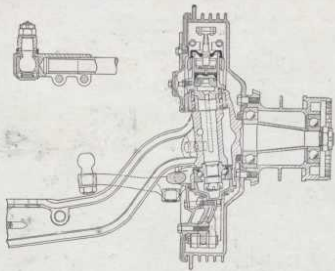
L'essieu avant présente plusieurs caractéristiques intéressantes. Le système de freins hydrauliques Duesenberg n'utilise qu'un seul piston placé verticalement, ce qui réduit les chances de fuite et empêche que la boue et les poussières n'atteignent le piston en caoutchouc. Aucun réglage n'est nécessaire au talon des sabots de frein, le point d'attaque est si judicieusement choisi que tout réglage est superflu. Par suite, le seul réglage à effectuer est le rattrapage de l'usure de la garniture et les deux sabots sont réglés en même temps comme il est montré. Pour effectuer le réglage, amener le sabot avant en contact avec le tambour sans toucher pour le moment au sabot arrière ; dès que l'on agit pour la première fois sur la pédale de frein, le mécanisme réajuste automatiquement le jeu uniformément entre les deux sabots, la liaison compensatrice étant montée sur un pivot libre.
